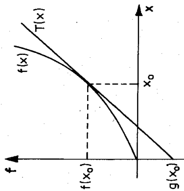
Zur Legendre-Transformation
